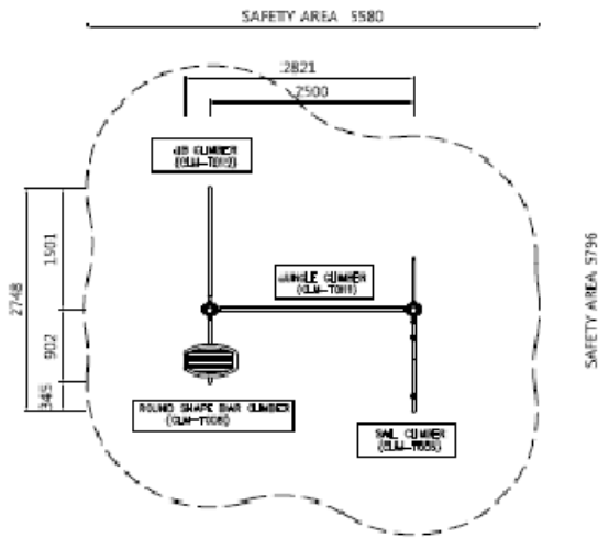
Layout Drawing Scale: 1:none
